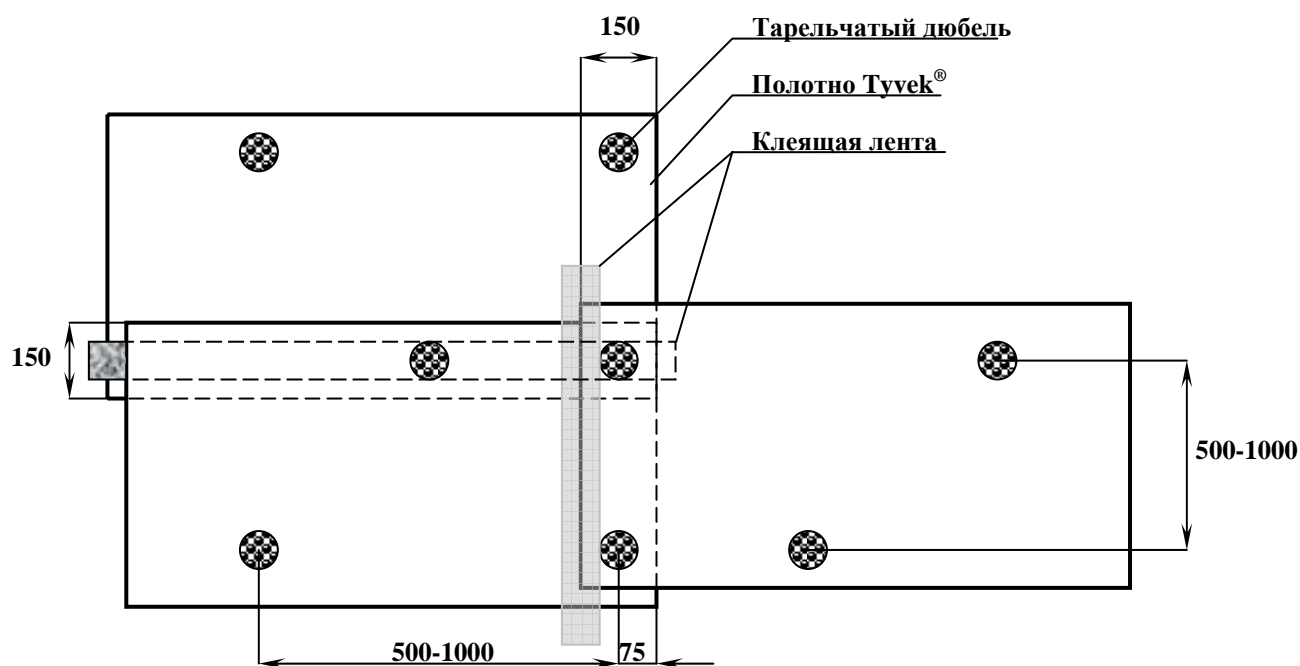
СХЕМА ЗАКРЕПЛЕНИЯ МАТЕРИАЛА «Tyvek®»
