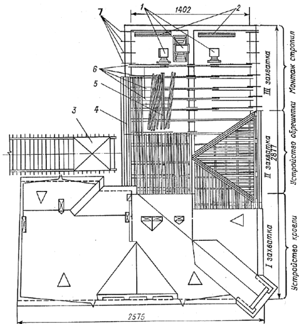
Рис.8. Схема организации работ по монтажу дощатых стропил
