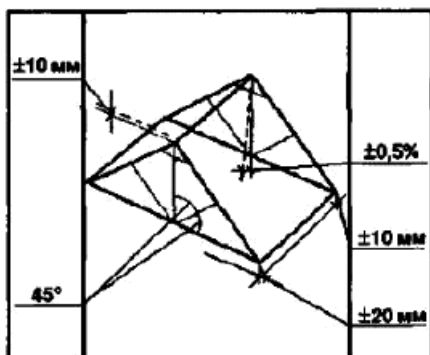
Рис.9. Допускаемые отклонения при монтаже стропильной системы
