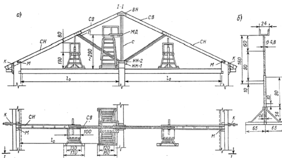
Рис.6. Монтажная схема дощатой стропильной фермы
