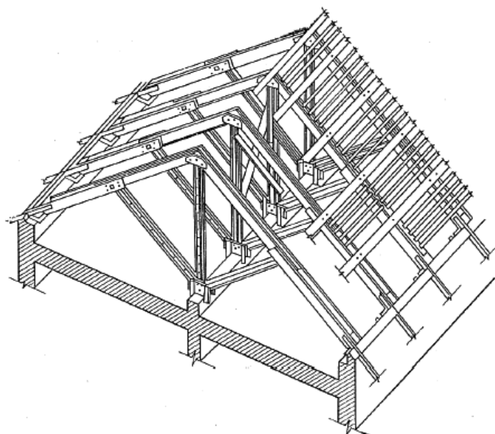
Рис.7. Общий вид сборных дощатых стропил
