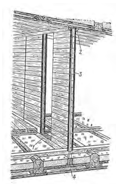
Рис.16. Схема установки дощатой щитовой перегородки
