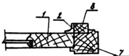
Рис.15. Узел оформления выступающих углов перегородок угловыми стойками
