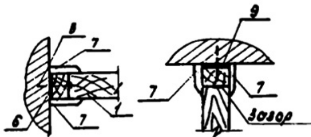
Рис.11. Узлы крепления щитов к стенам и потолкам
