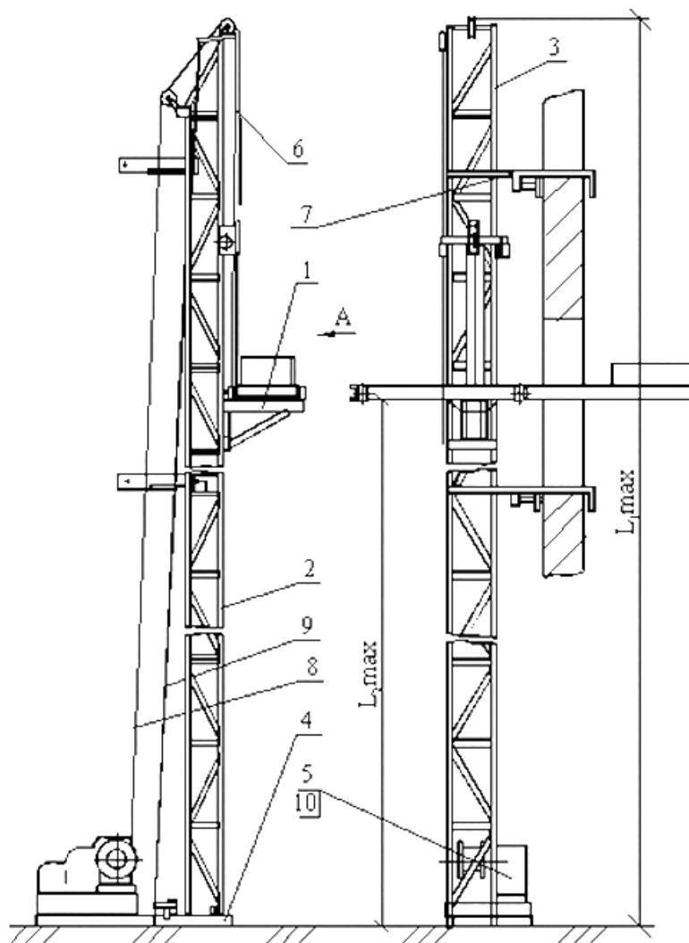
Рис.6. Схема монтажа мачтового подъемника
