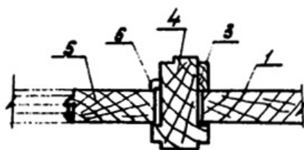
Рис.12. Узел навески двери в перегородке к промежуточным стойкам
