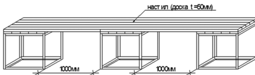
Рис.8. Установка подмостей в рабочее положение
