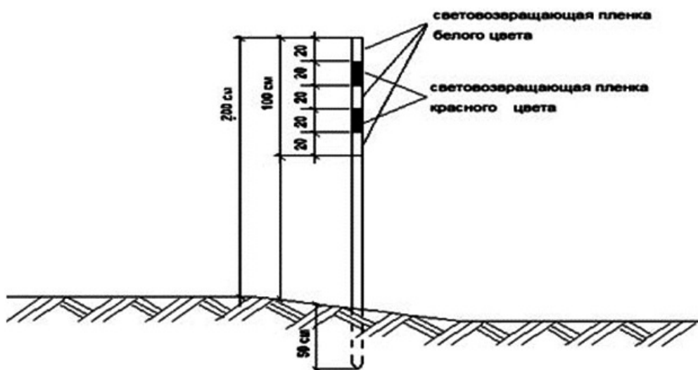
Рис. 2. Схема установки указательной вехи
