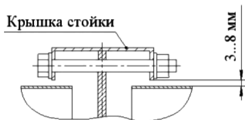
Рисунок 12 - Установка крышки стойки
