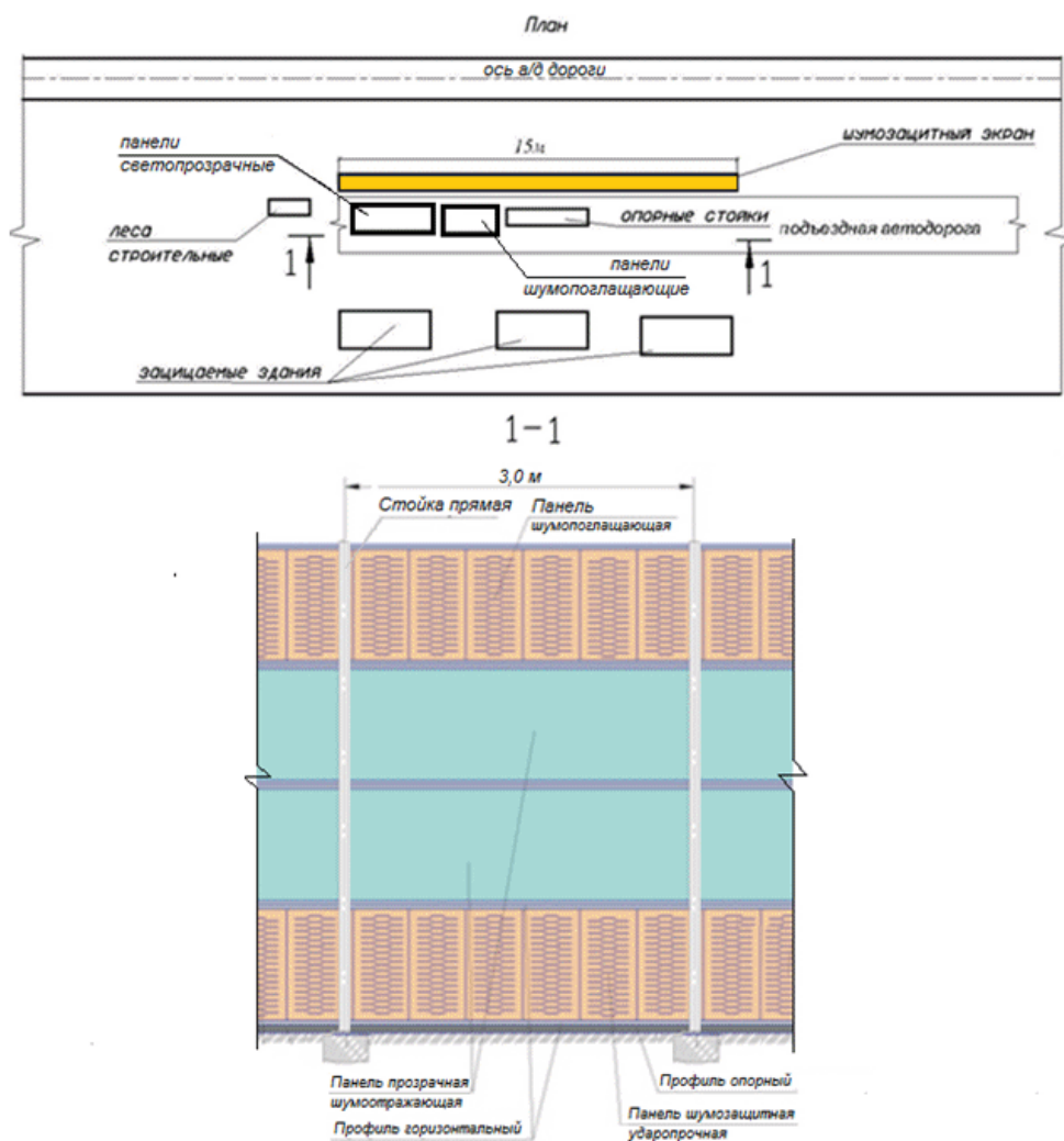
Рисунок 3 - Организация рабочей зоны
