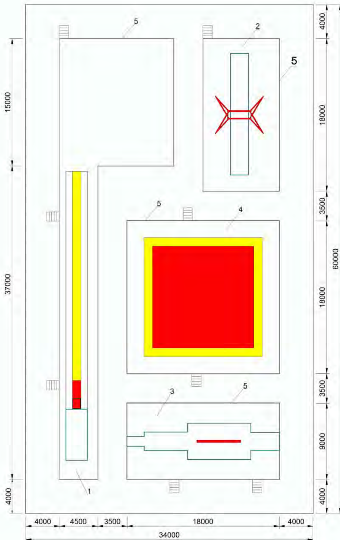
1 – зона опорного прыжка; 2 – зона упражнений на разновысоких брусьях; 3 – зона снаряда «бревно»; 4 – площадка для вольных упражнений; 5 – помост / граница зоны безопасности
