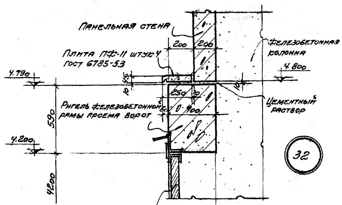
Ворота распашные 4000 x 4200 по сер. пр. 05-36.2
